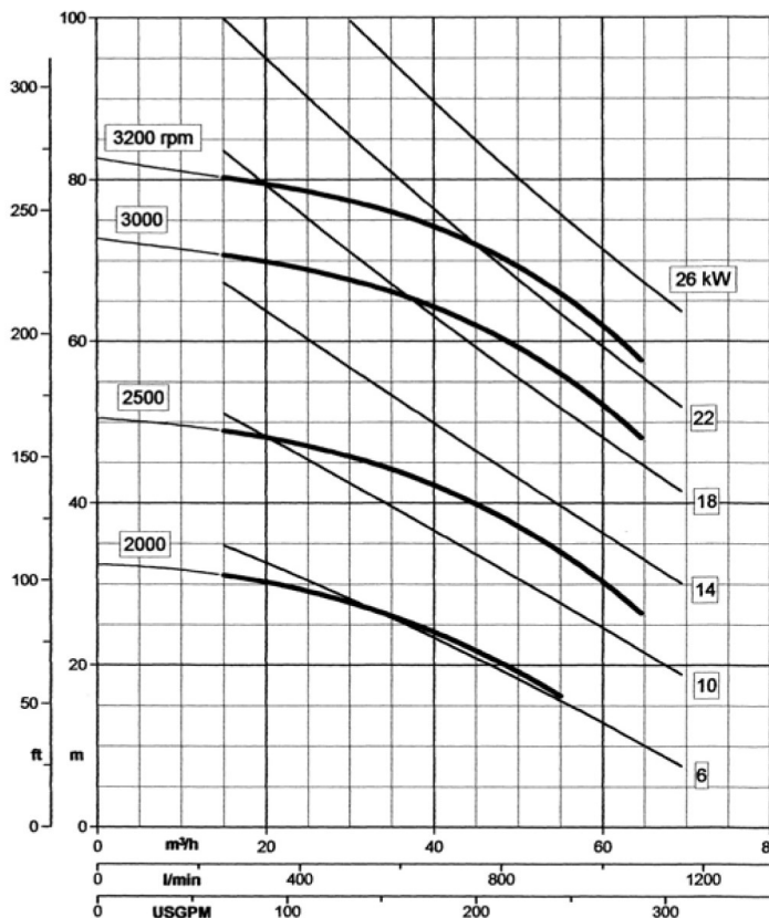
Curva con motore a 2900 rpm
