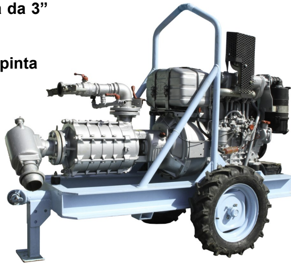
Motopompa Mod. GEO MP3_SH_SUN2015
