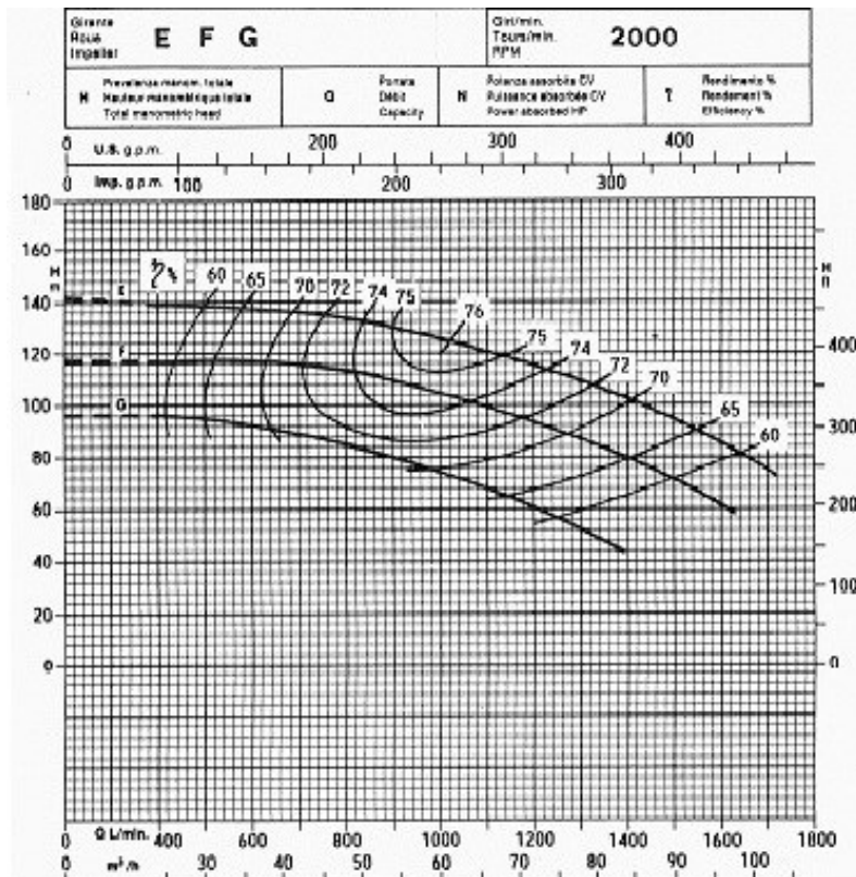
Curva con motore a 2000 rpm
