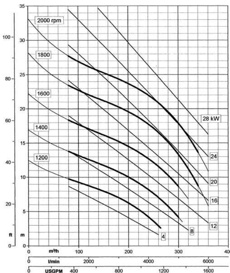
Motopompa Mod. GEO MP6 W
