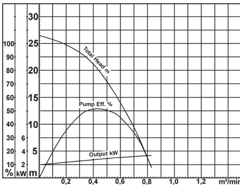
Curva con motore a 2900 rpm
