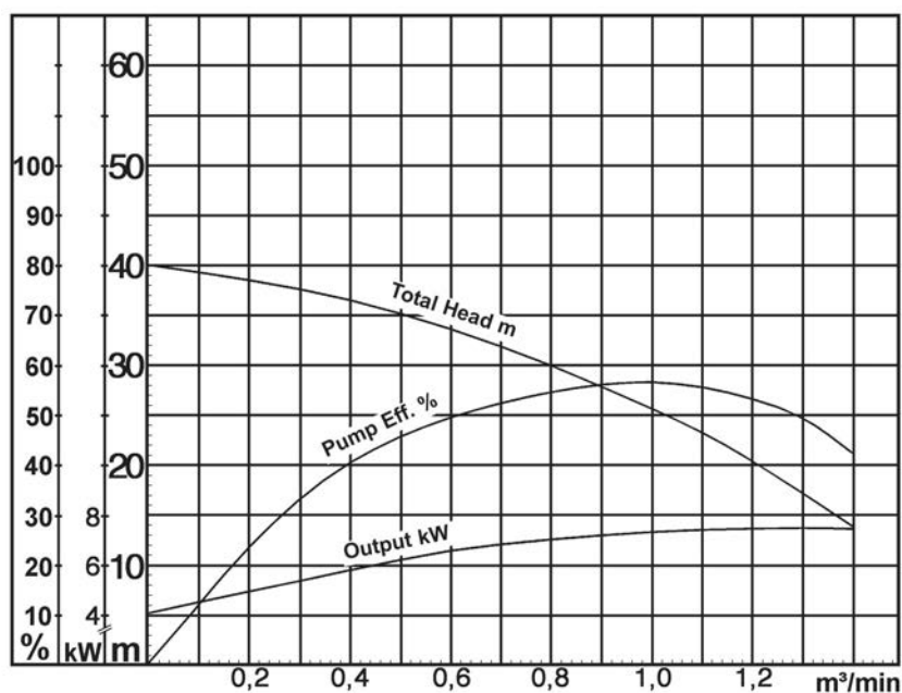
Curva con motore a 2900 rpm
