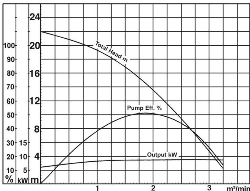
Curva con motore a 1450 rpm
