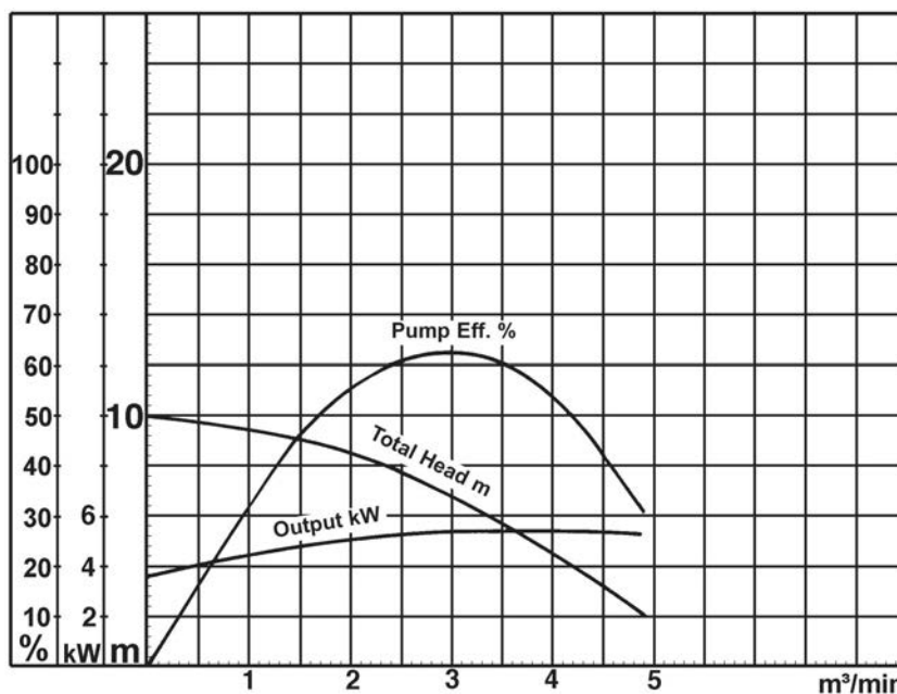
Curva con motore a 1450 rpm
